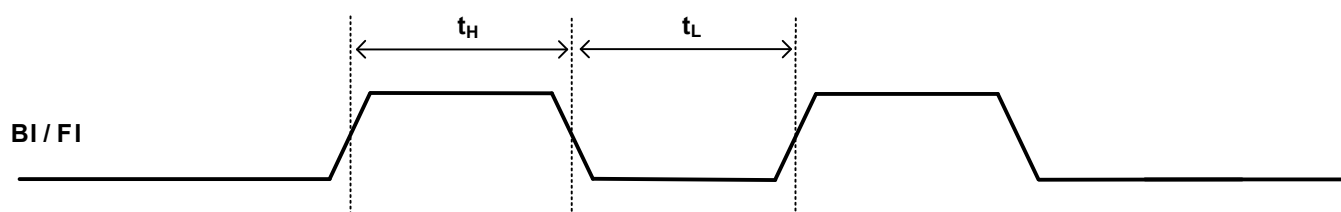
图 6. 上电时序图
