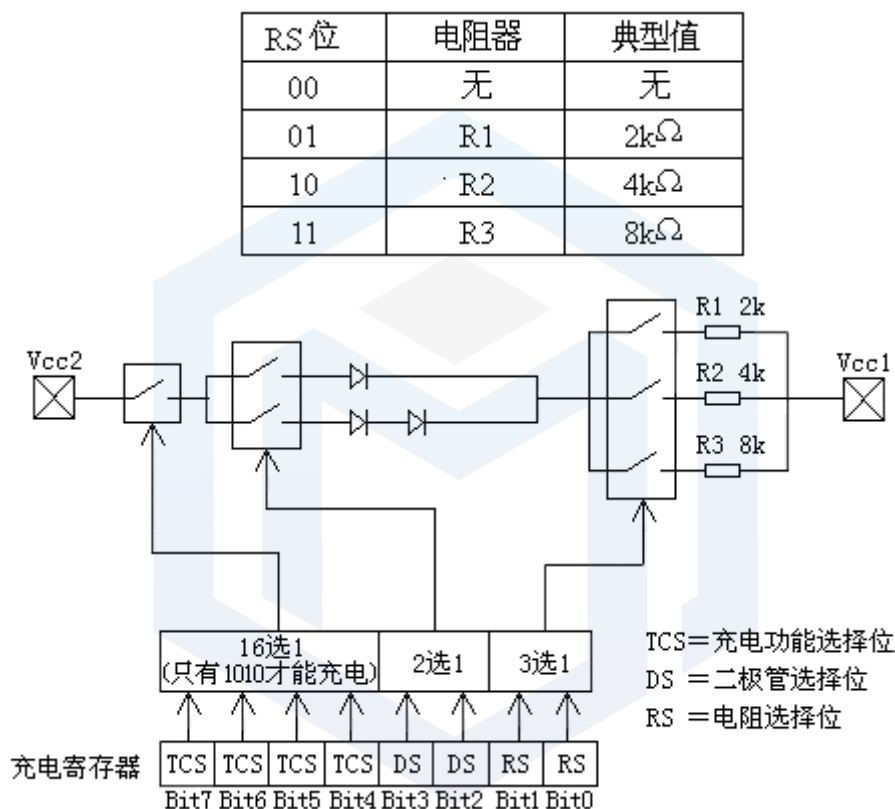
图 4 DS1302 可编程慢速充电器
